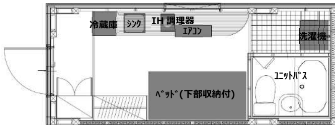
<客室図>
